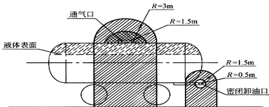
图 B.0.4 油罐车卸汽油时爆炸危险区域划分
