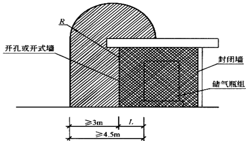
图 B.0.15 存放压缩天然气储气瓶组的房间爆炸危险区域划分
