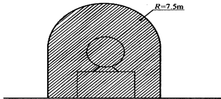
图 B.0.14 露天(棚)设置的天然气压缩机组、阀门、法兰或类似附件爆炸危险区域划分
