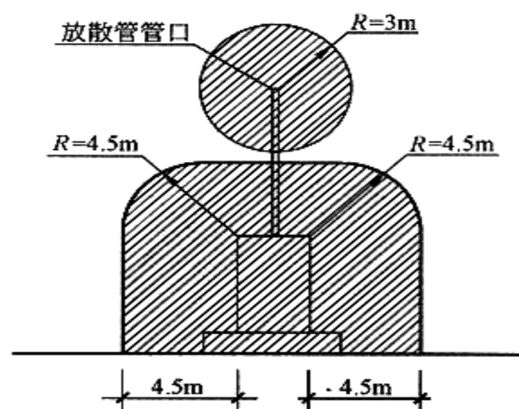
图 B. 0. 12 室外或棚内压缩天然气储气瓶组（储气井）爆炸危险区域划分
