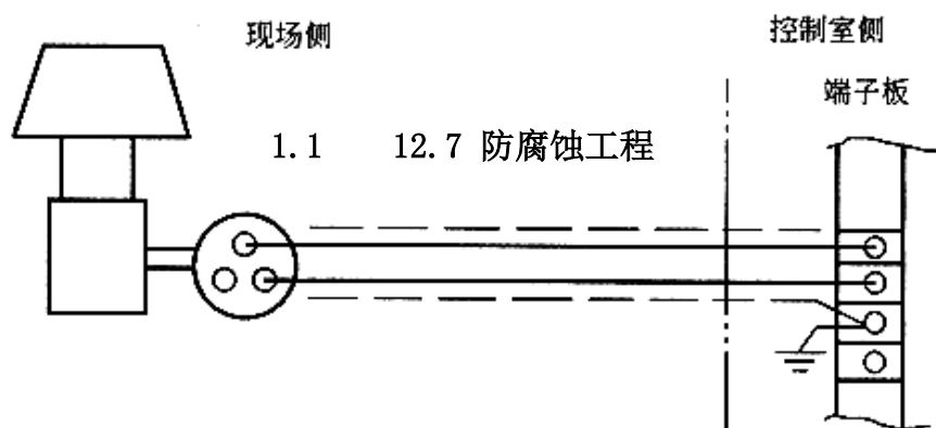
图 12.6.7 电缆屏蔽单端接地
