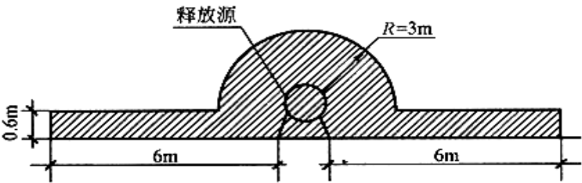
图 B.0.9 露天或棚内设置的液化石油气泵、压缩机、阀门、法兰或类似附件的爆炸危险区域划分
