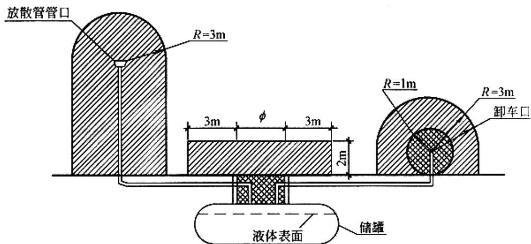
图 B.0.7 埋地液化石油气储罐爆炸危险区域划分
