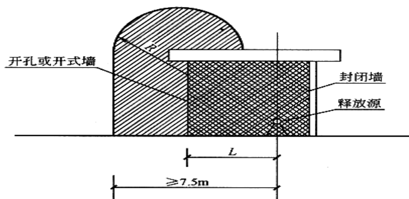
图 B. 0. 13 天然气压缩机、阀门、法兰或类似附件的房间爆炸危险区域划分 注： L \geq 4.5\text{m} 时， R = 3\text{m} ； L < 4.5\text{m} 时， R = 7.5 - L 。
