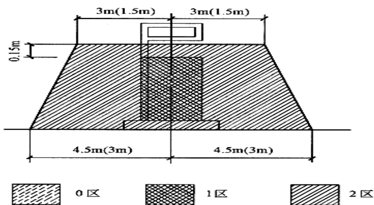
图 B. 0.3 汽油加油机爆炸危险区域划分
