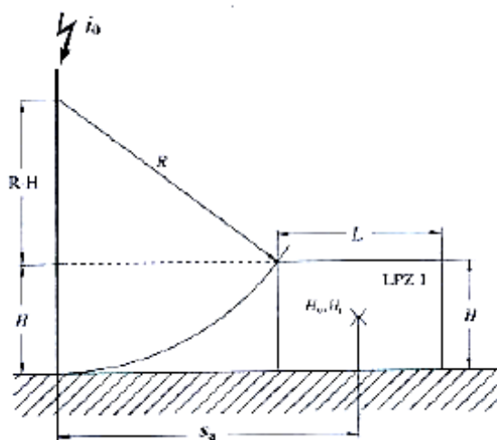
图 6.3.2-2 取决于滚球半径和建筑物尺寸的最小平均距离
