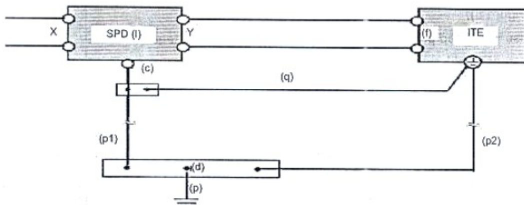
图 J. 2. 4-2 将多接线端子电涌保护器的有效电压保护水平
