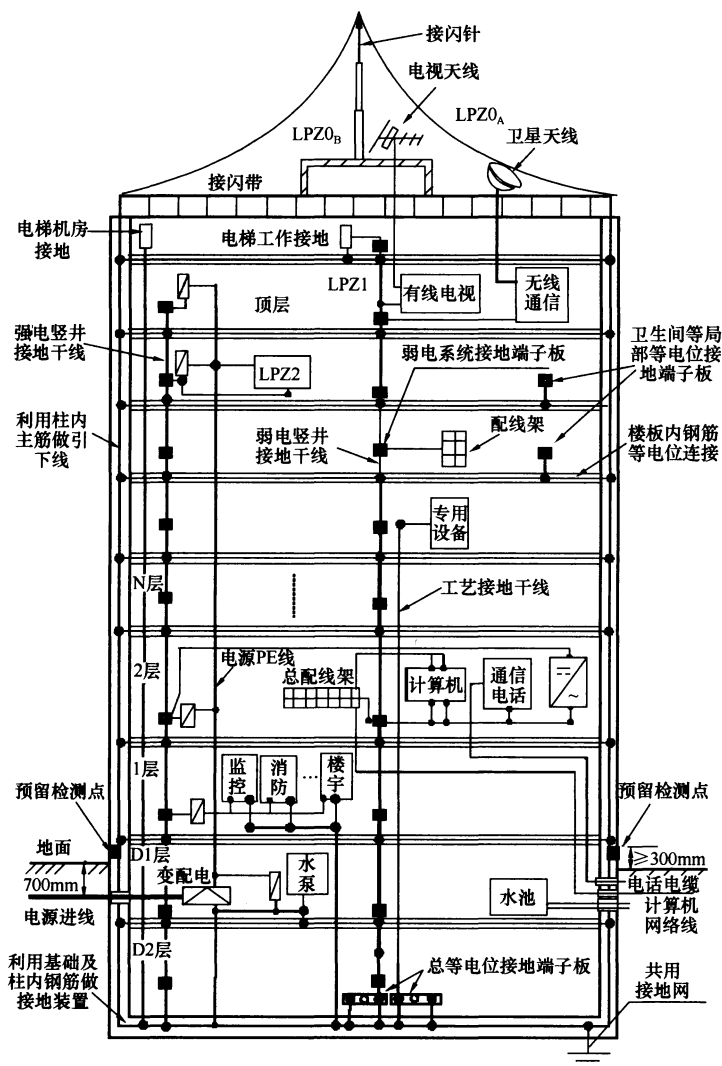
图 6 建筑物等电位连接及共用接地系统示意图
