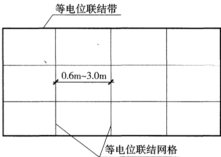
图 3 等电位联结带与等电位联结网格
