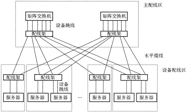
图 12 前端网络布线系统基本结构图(三)
