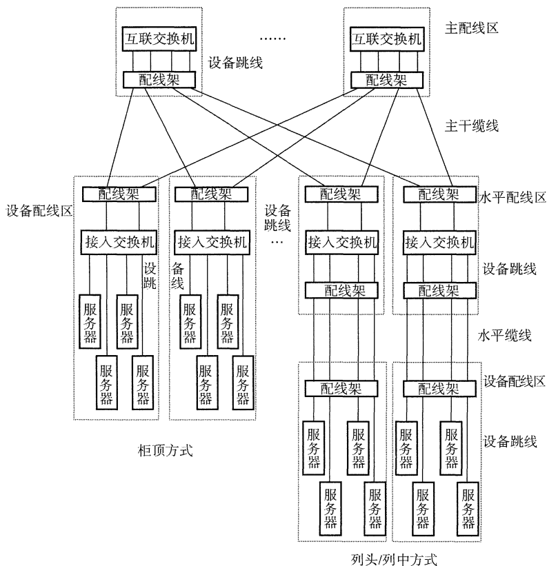
图 11 前端网络布线系统基本结构图(二)
