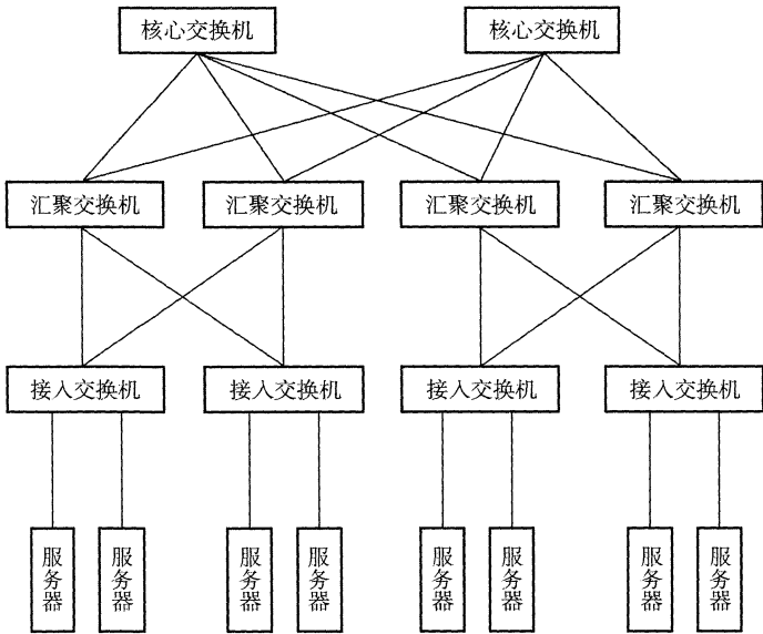
图 5 数据中心三层网络架构图
